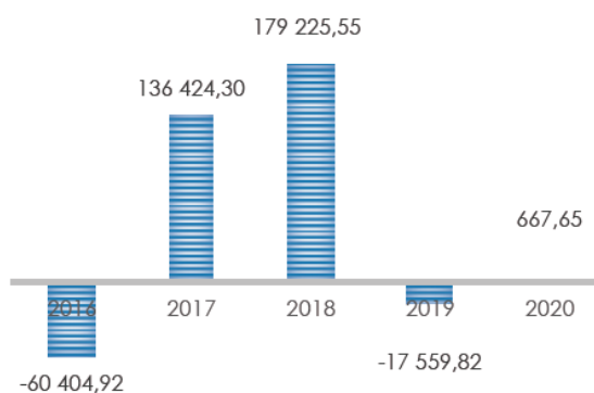
Gráfico 7 :: Resultado líquido
