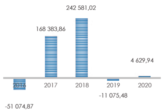
Gráfico 6 :: EBITDA
